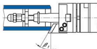
Удаление сварного шва между трубой и трубной решеткой
